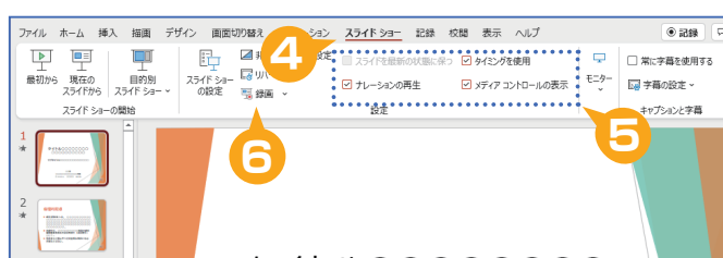
図4. 録音の設定
